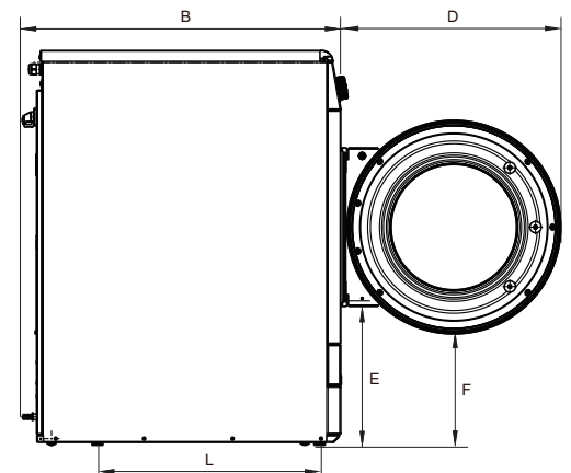
Lato sinistro
