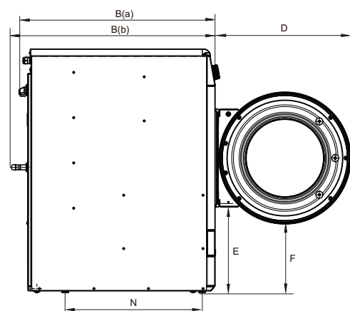
Lato sinistro
